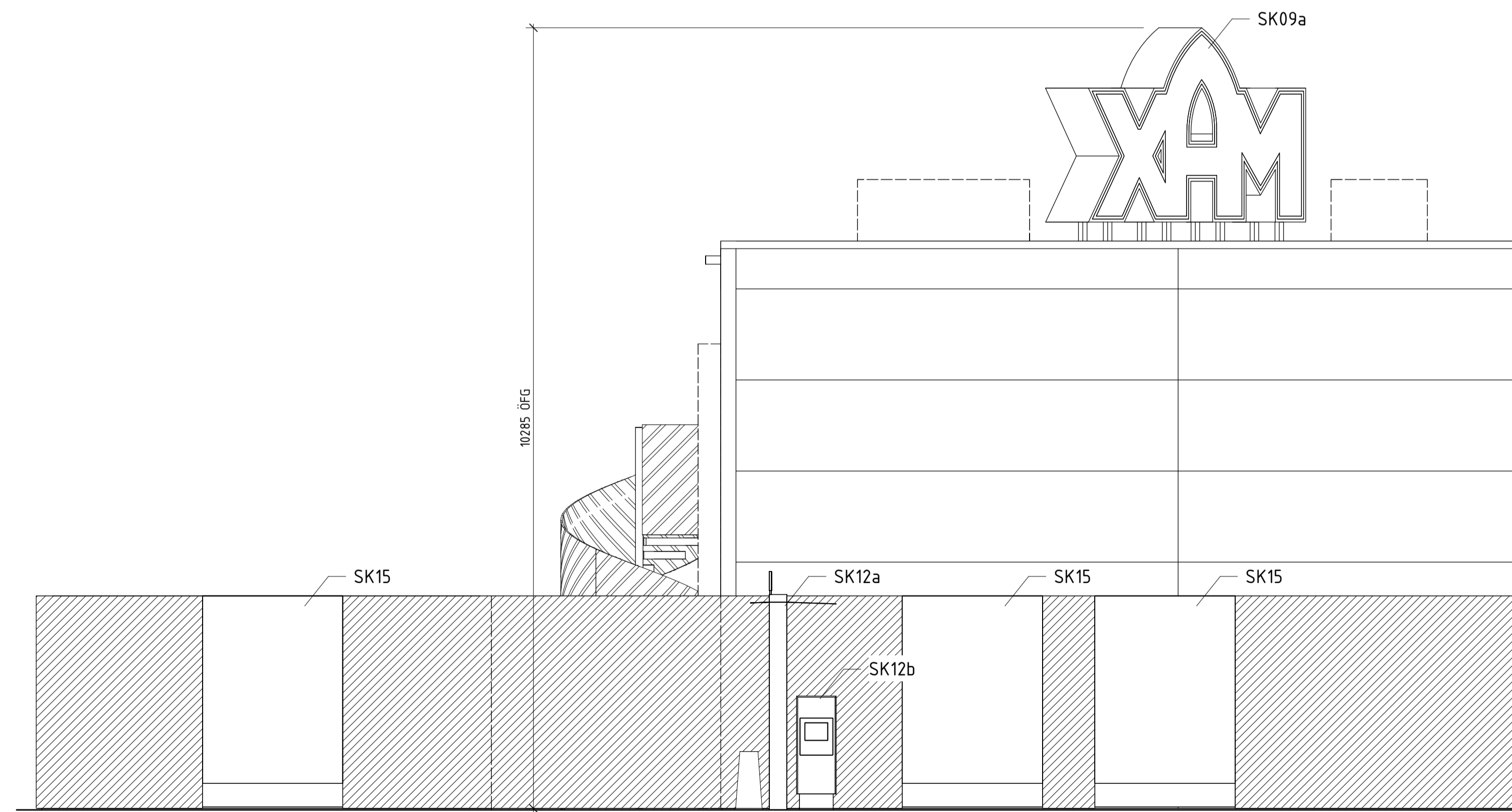
FASAD MOT DRIVE DEL 2
