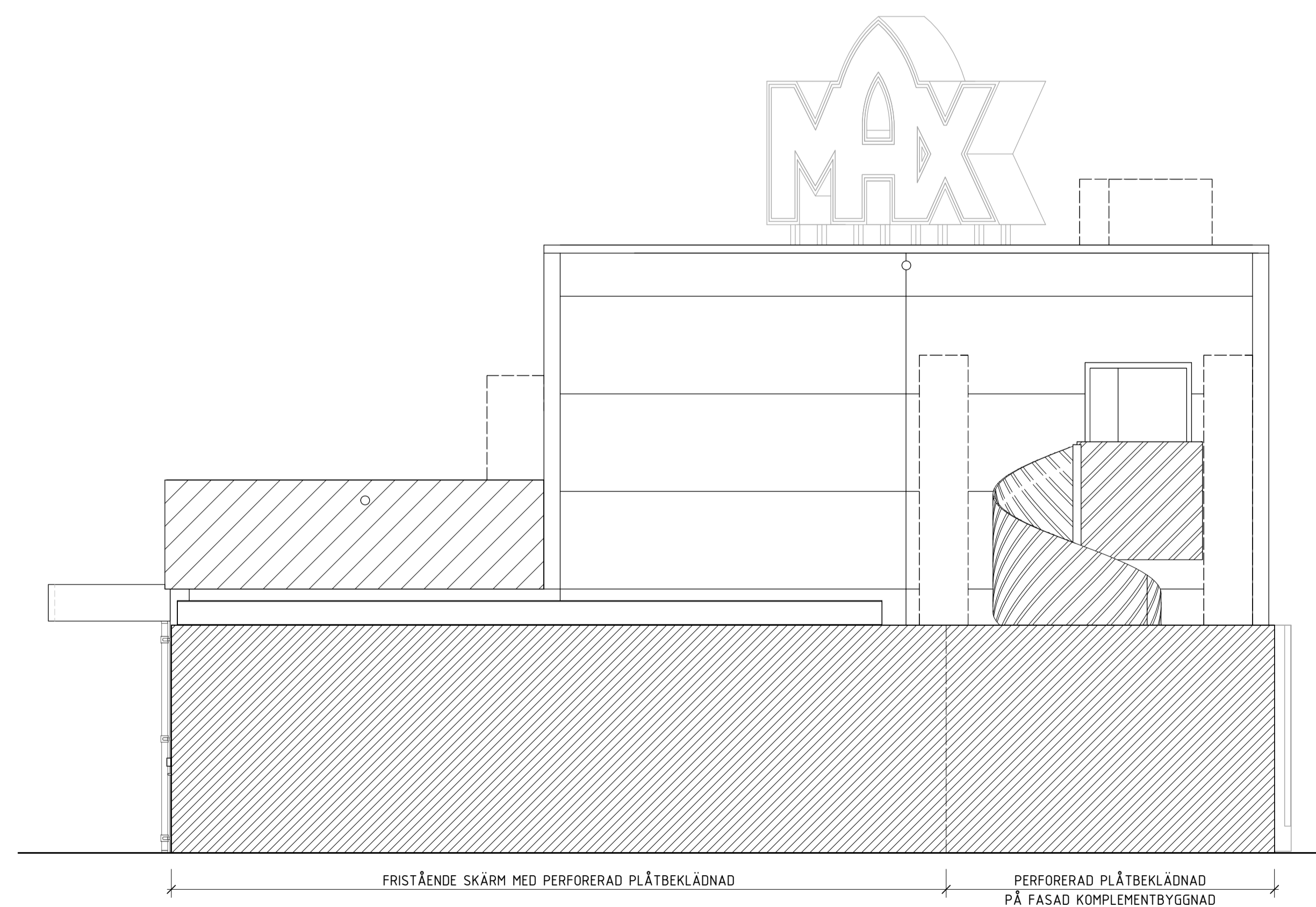
FASAD MOT LASTGÅRD MED SKÄRM
