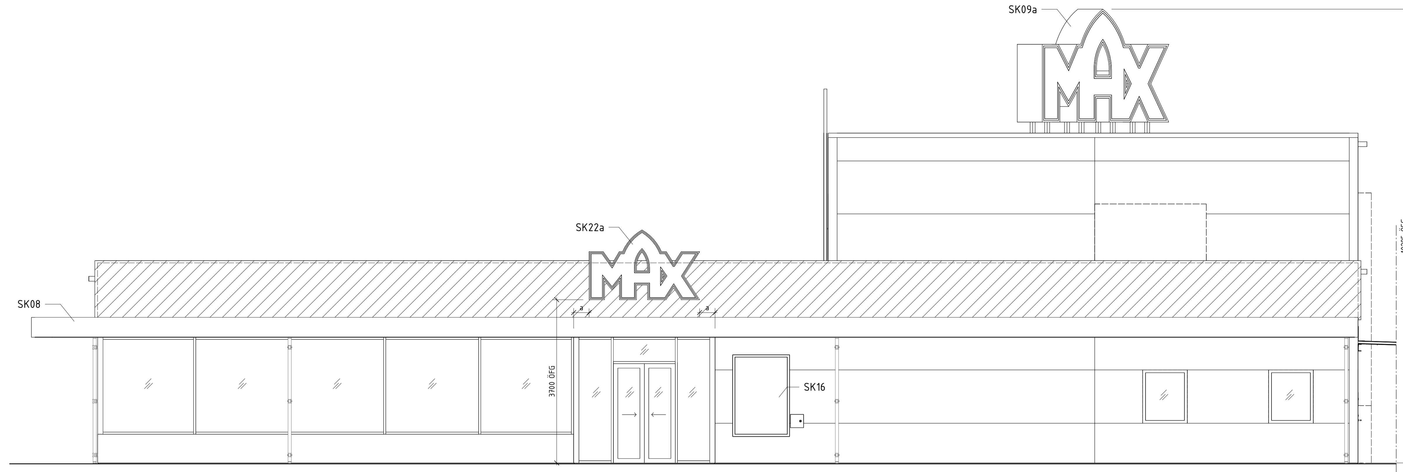
FASAD MOT ENTRÉ
