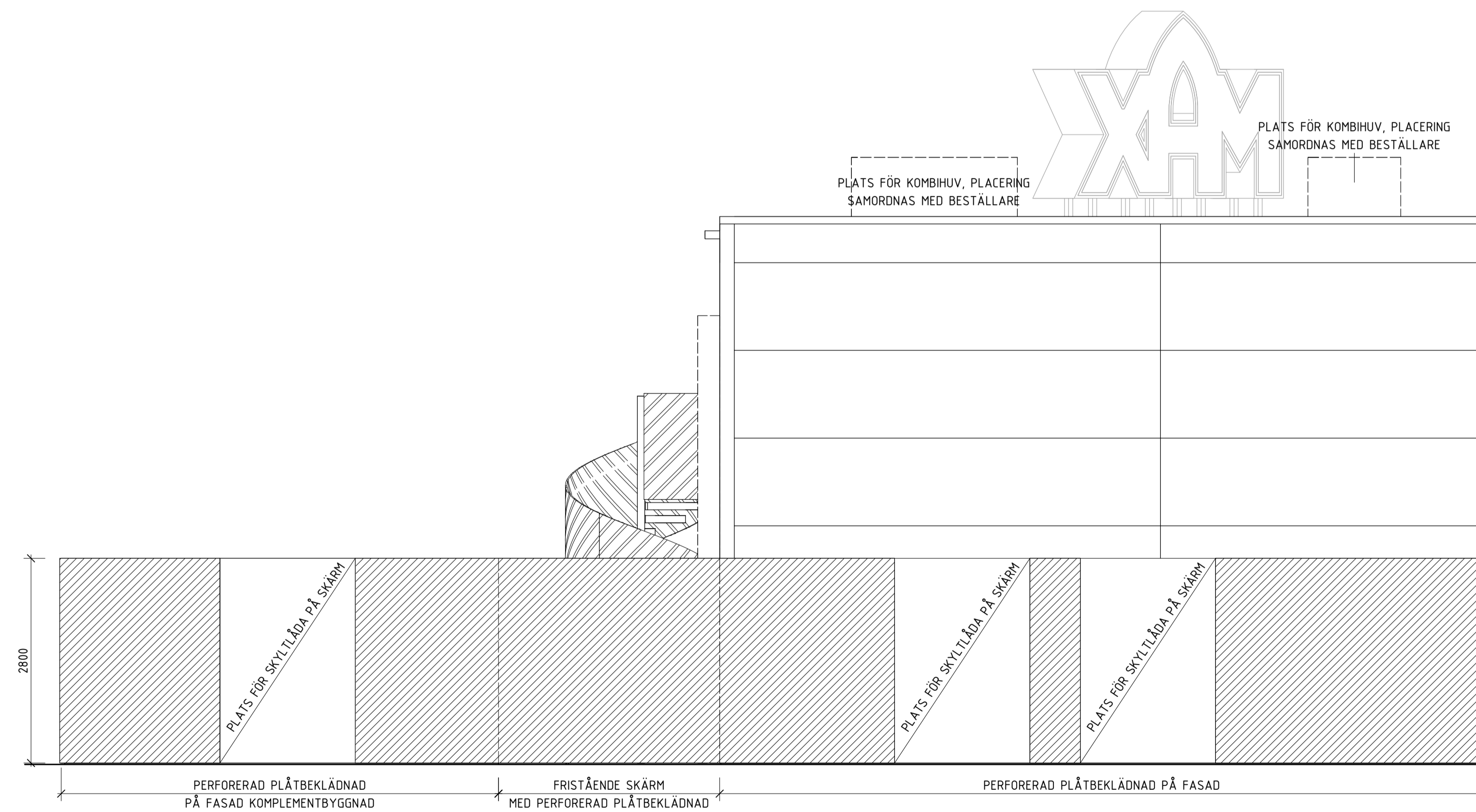
FASAD MOT DRIVE DEL 2
