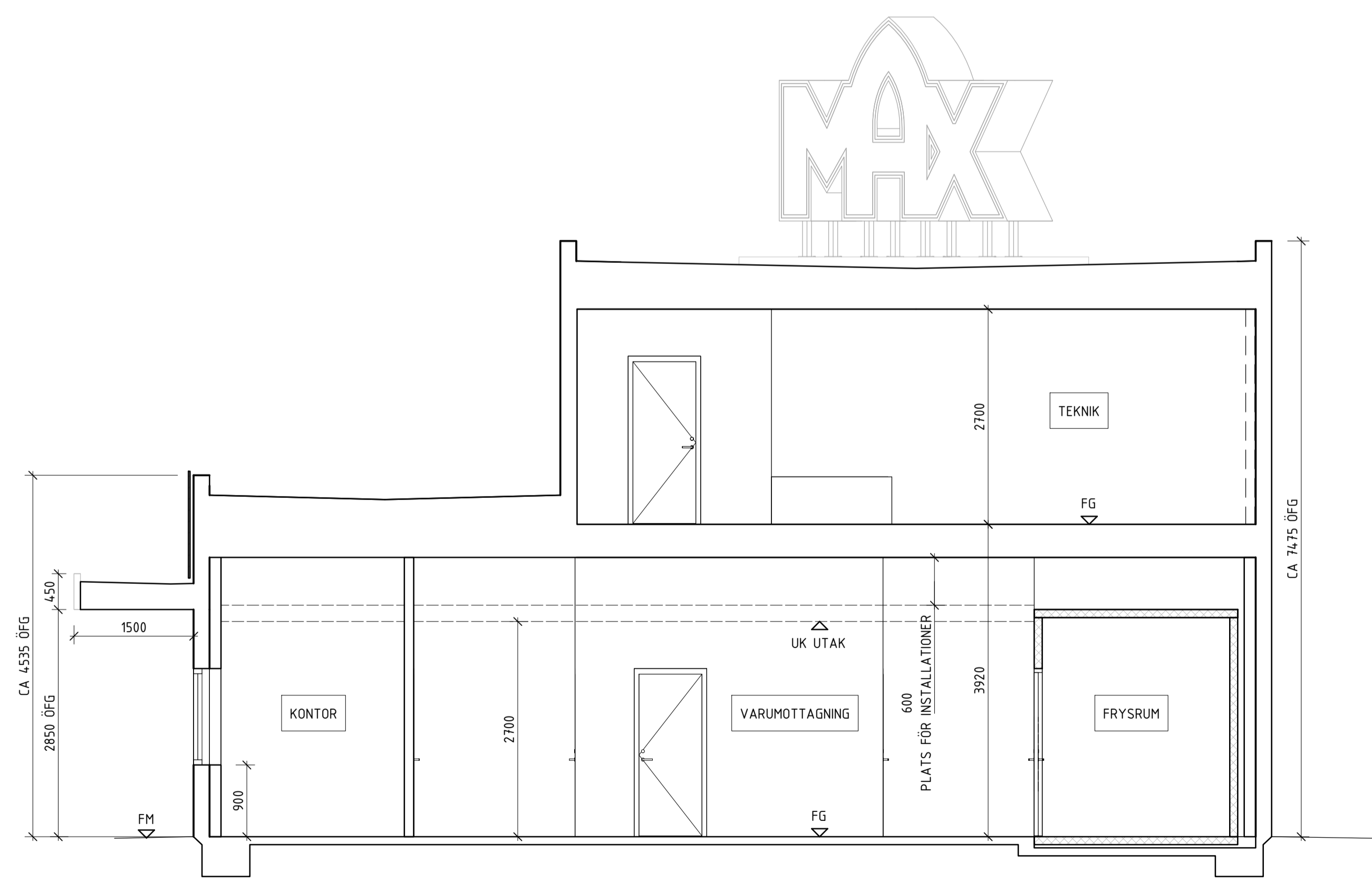
TVÄRSEKTION B-B
