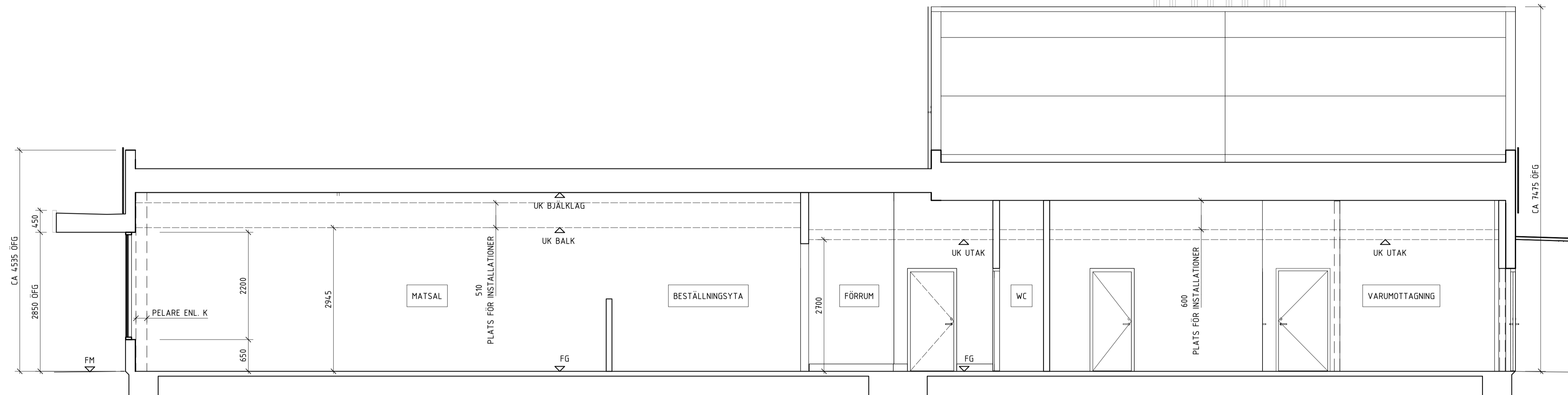
LÄNGDSEKTION A-A
