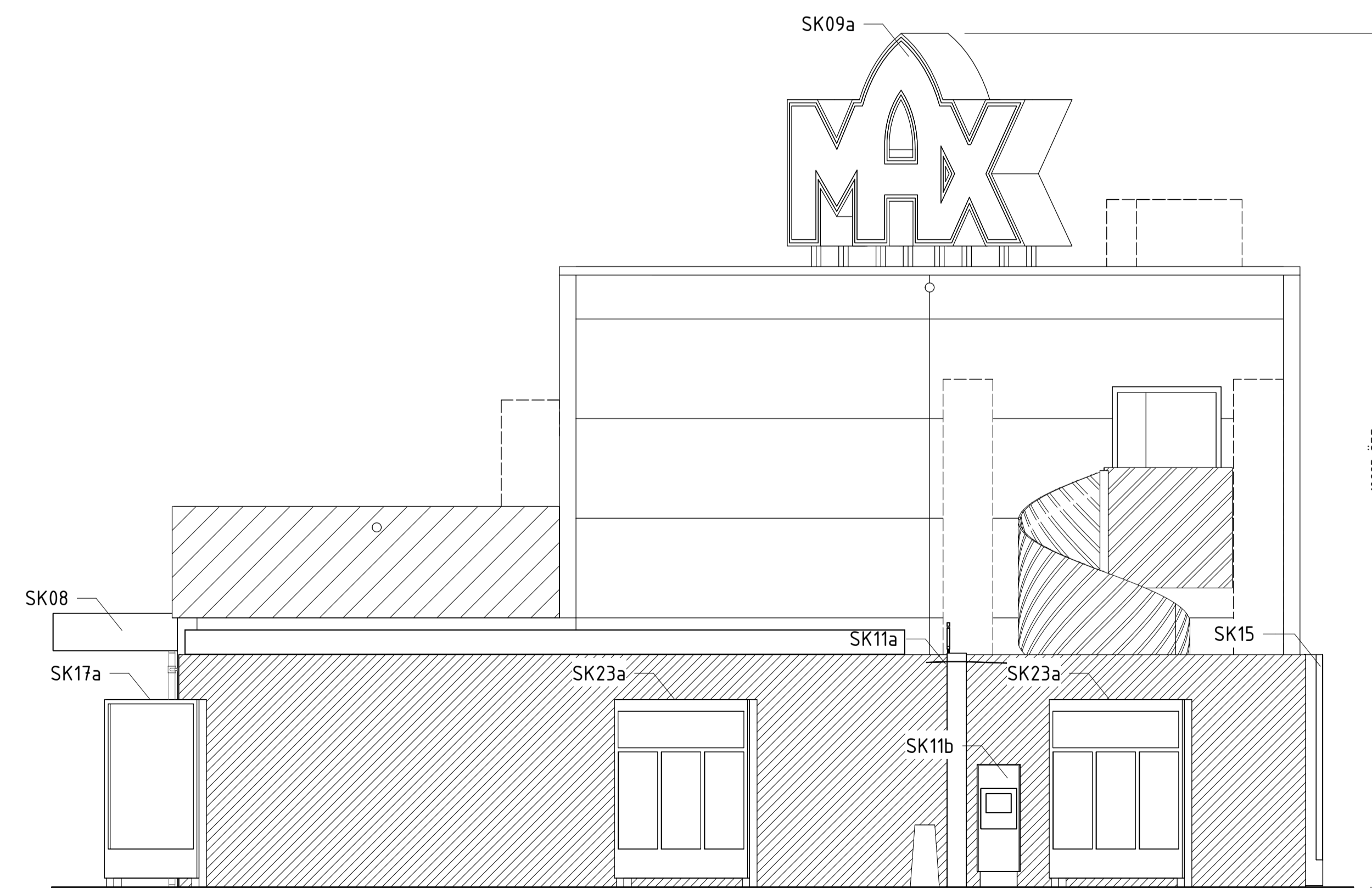
FASAD MOT LASTGÅRD MED SKÄRM
