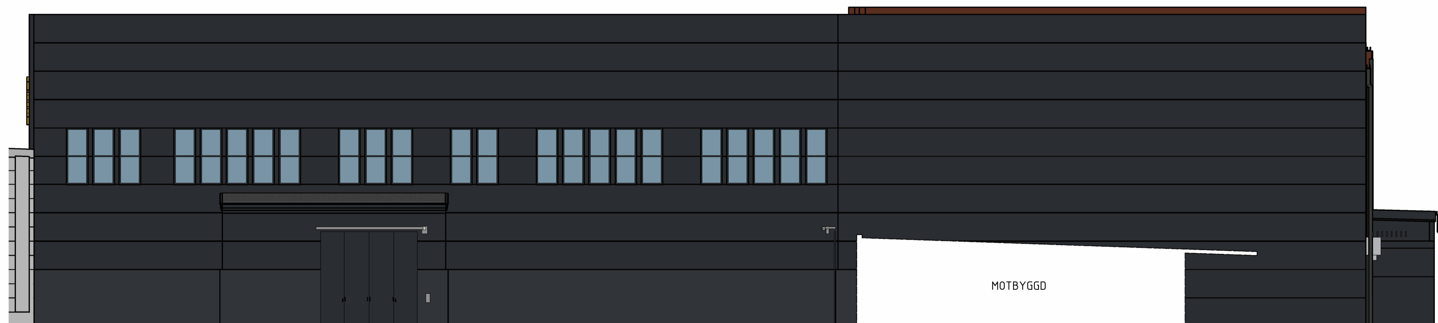
DELFA SAD MOT NORDVÄST 1 : 100
