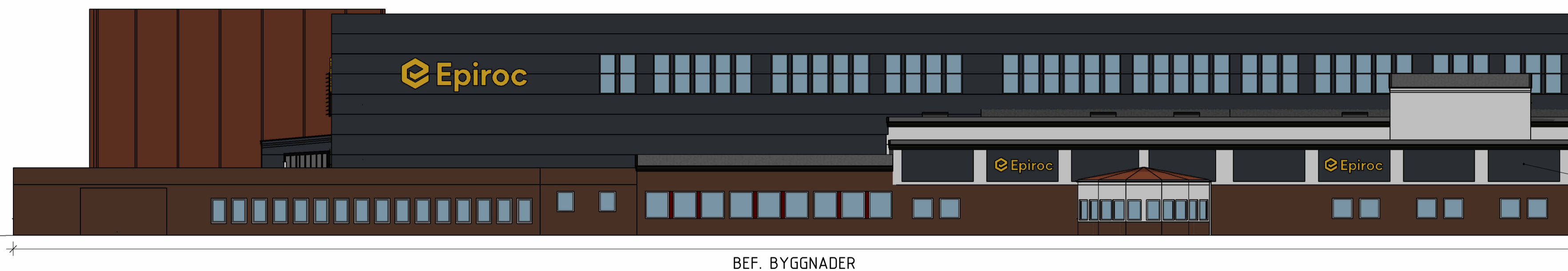
FASAD MOT NORDÖST, del A 1 : 200
